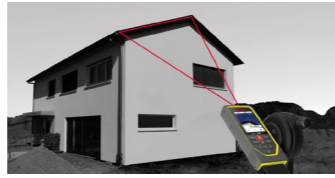
立面测量
